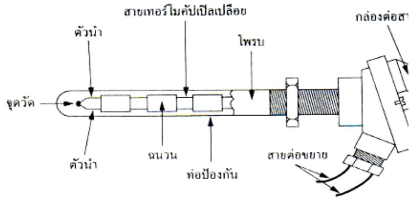
รูปแสดงโครงสร้างของเทอร์โมคัปเปิล
