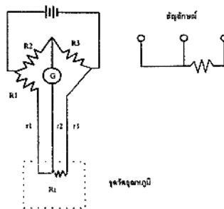
รูปที่ 2 แสดง RTD 3 สาย
